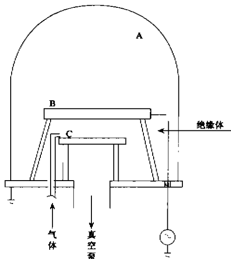
图1 等离子体发生装置示意图(A——真空室, B——正电极, C——基电极)
