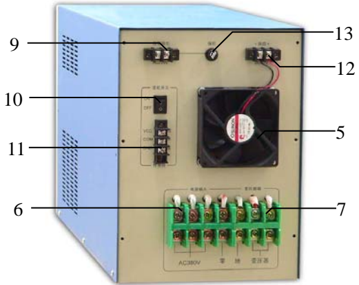
图 2、主机背板
