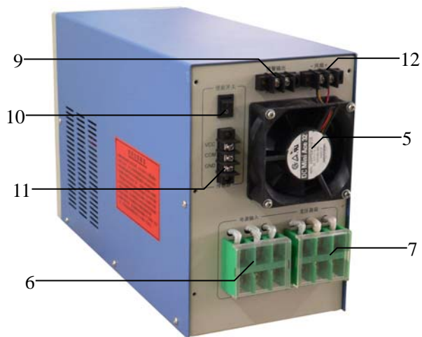
图 2、主机背板
