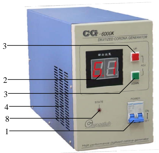
图 1、主机面板
