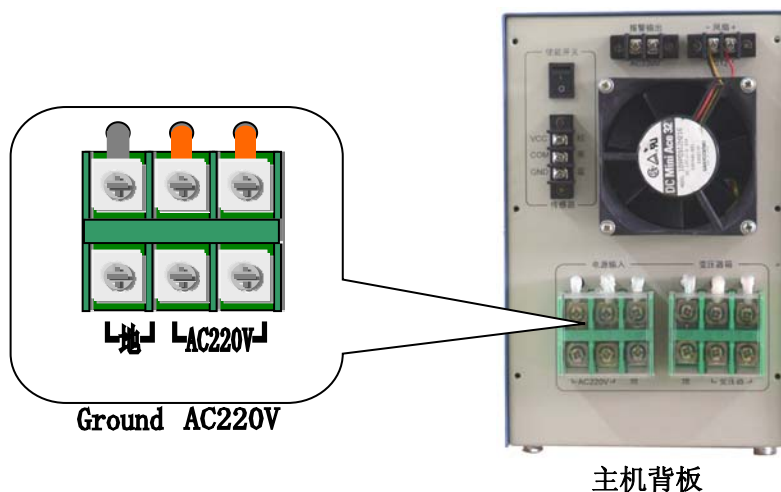
图 6、主机和 AC220V 电源的连接
