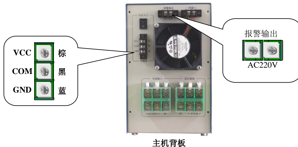
图 7、主机和传感器、报警的连接
